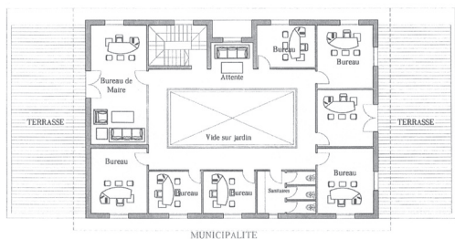
PLAN ETAGE
