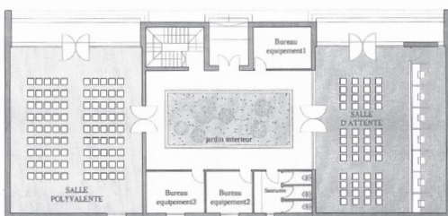
PLAN REZ-DE-CHAUSSEE
